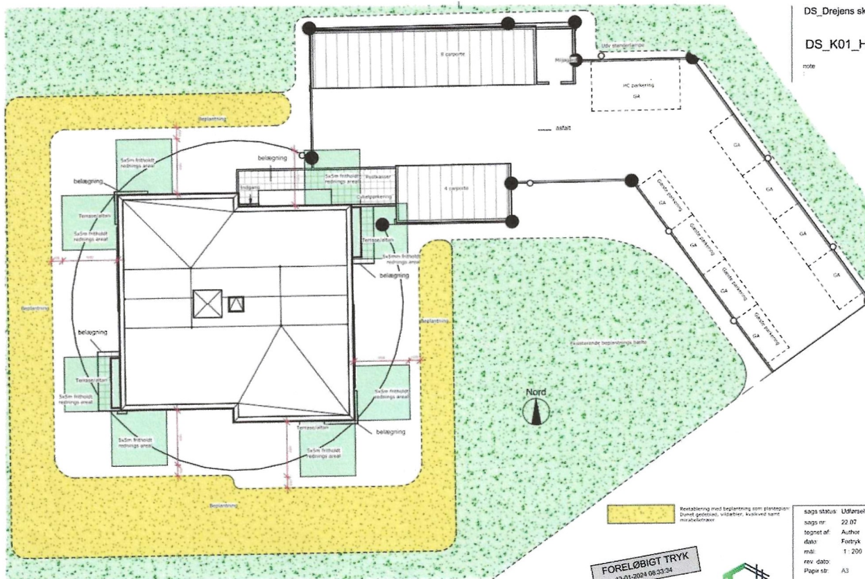
1 Anlægs plan princip 1 : 200
